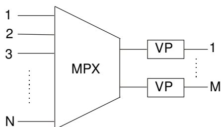
Obr. 3. Multiplexor s výstupným radením Fig. 3. Output queuing multiplexor
