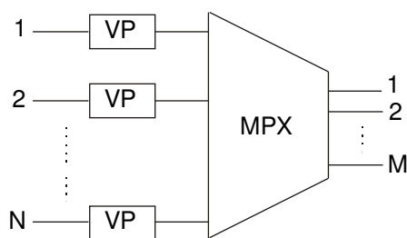
Obr. 2. Multiplexor so vstupným radením Fig. 2. Input queuing multiplexor
